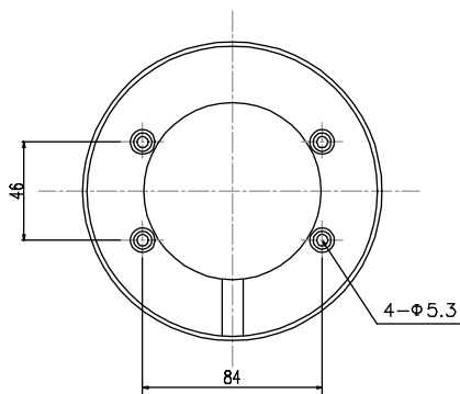
取付穴図
